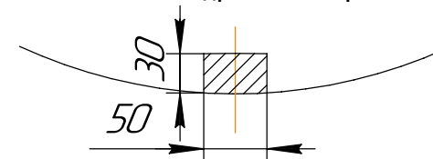
Эскиз подрезки бампера
